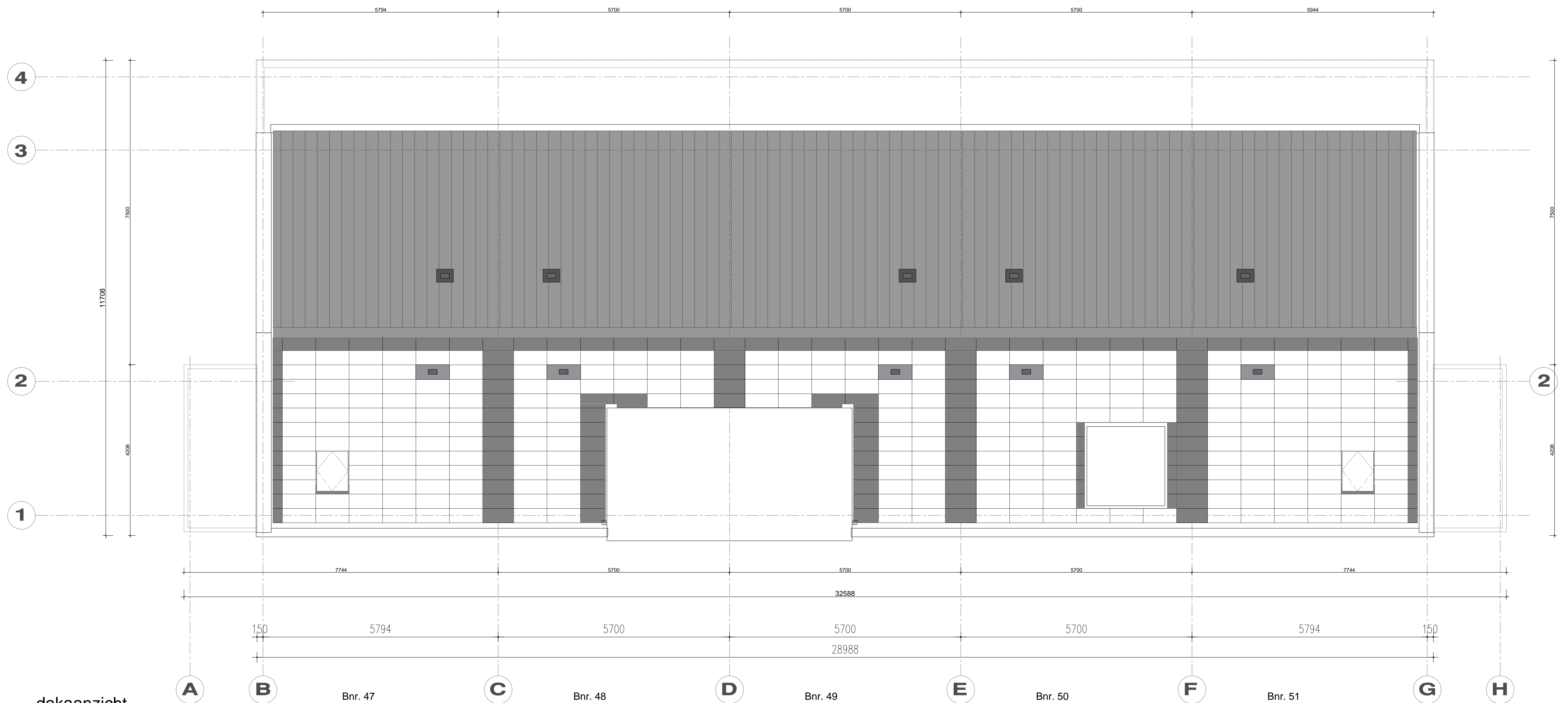
dakaanzicht 1 : 50
